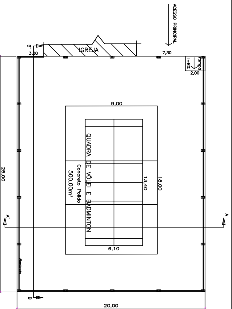
PLANTA BAIXA TÉCNICA 1/100
